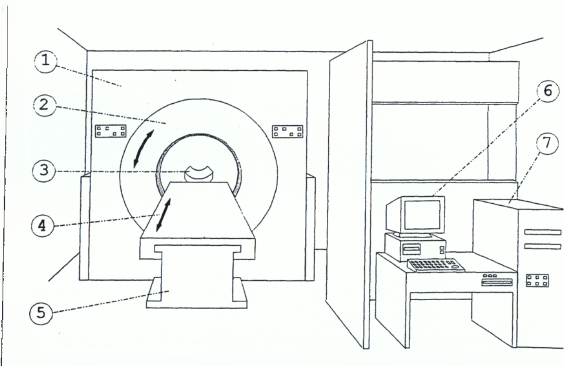
ΕΙΚΟΝΑ 1 : Γενική Διάταξη Αξονικού Τομογράφου
