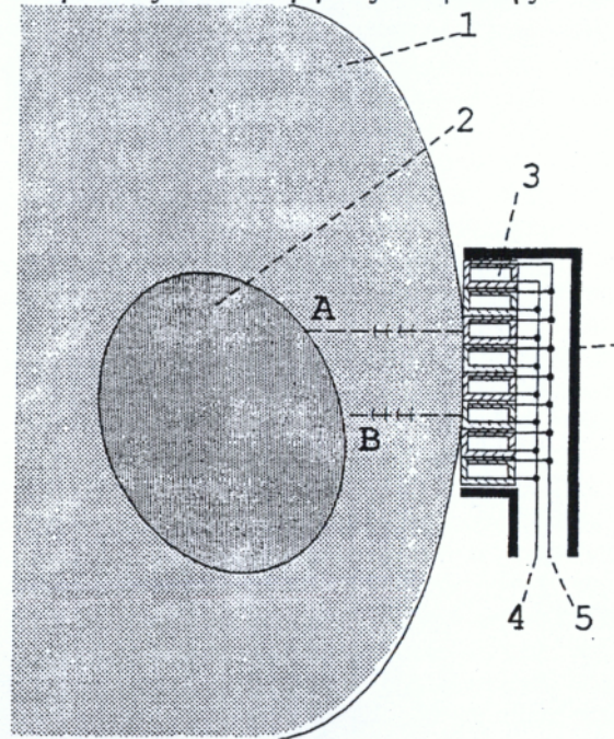
ΕΙΚΟΝΑ 3 : Τρόπος Λειτουργίας Κεφαλής Υπερηχογράφου
