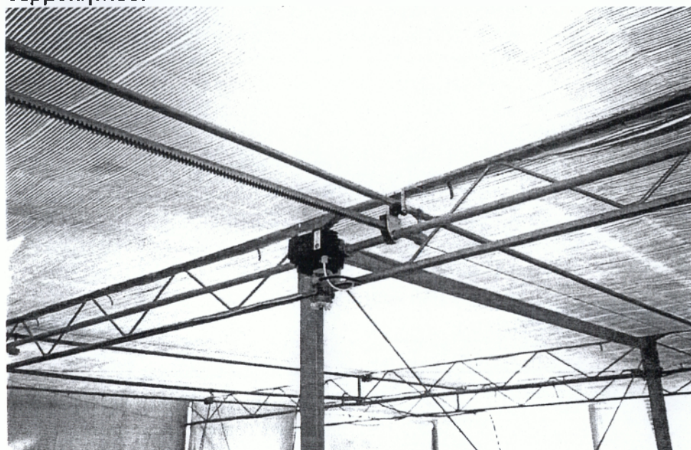
Εικόνα 2. Μηχανισμός ρύθμισης των θερμοκουρτινών
