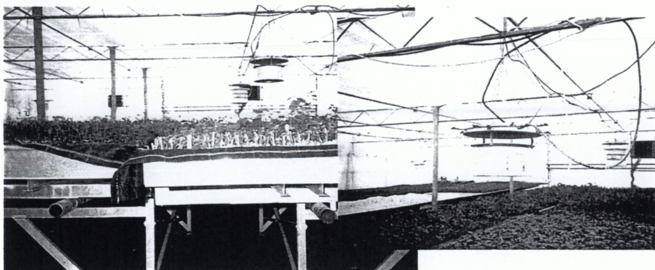
Εικόνα 7. Τραπέζια καλλιέργειας με μεταλλικό σκελετό και κυλιόμενη επιφάνεια. Εικόνα 8. Ψεκαστήρες πάνω από τα Τραπέζια καλλιέργειας
