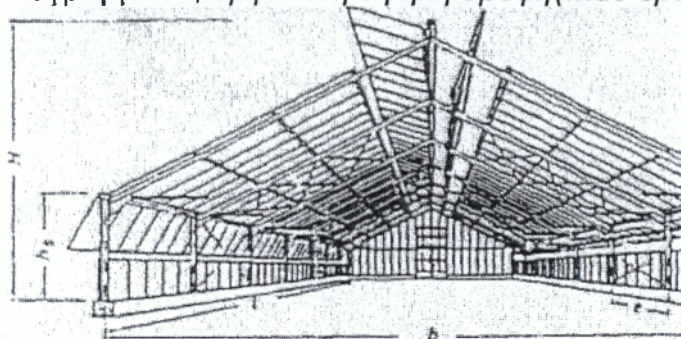
Διάγραμμα 19, αμφικλινή χαμηλή οροφή ( venlo )
