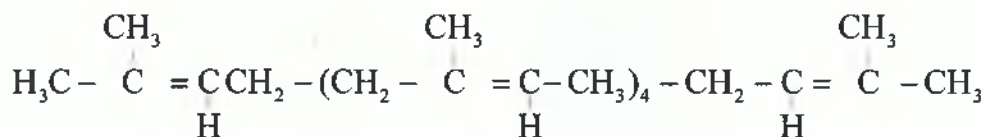
Σχήμα 4.2 Σκουαλένιο
