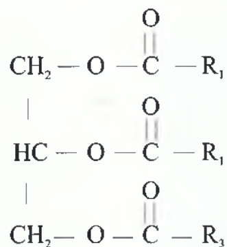
Σχήμα 4.1: Τριγλυκερίδιο
