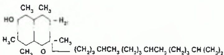
Σχήμα 4.5 α-Τοκοφερόλη
