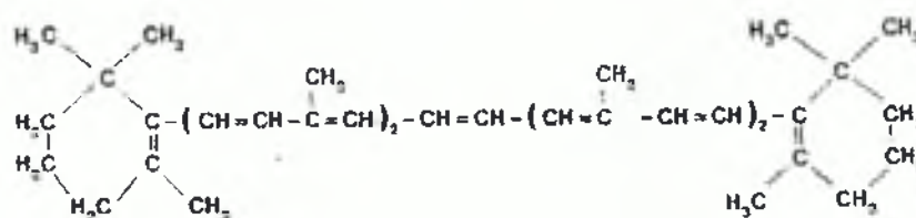
Σχήμα 4.6 β-Καροτίνη
