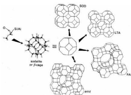
Εικόνα 12: Δόμη Ζεολίθων (Καλάρης, 2016)
