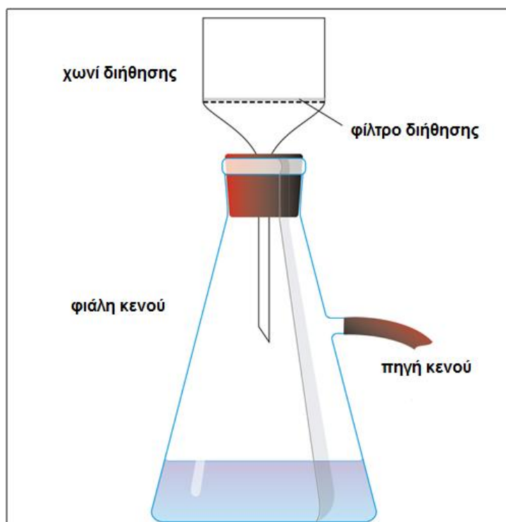
Εικόνα 15: Η φιάλη διήθησεως υπό κενό Büchner και τα μέρη της (Anon., 2014)
