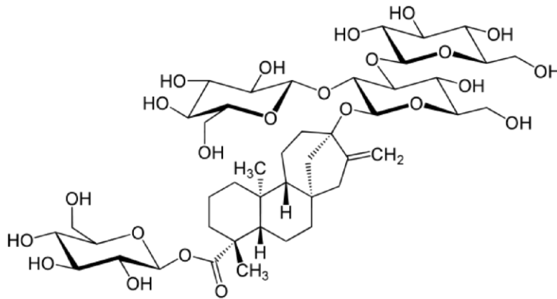
Εικόνα 7: Δομή ρεμπαουδιοσίδη A (rebudioside A)
