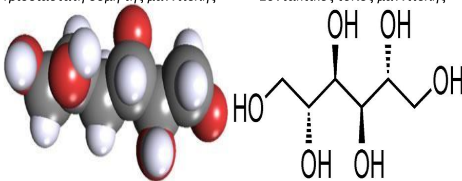
Εικόνα 13: Τρισδιάστατη δομή της μαννιτόλης (αριστερά), Συντακτικός τύπος μαννιτόλης(δεξιά) (wikipedia, 2016)
